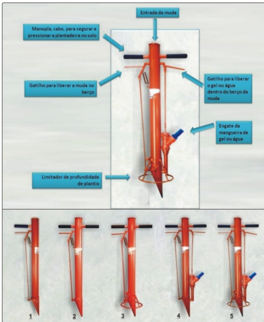
Figura 10 – Modelos comerciais de plantadeiras manuais com e sem aplicadores de gel e/ou água; com e sem limitador de profundidade. (Fotos cedidas pela Catec Equipamentos).
