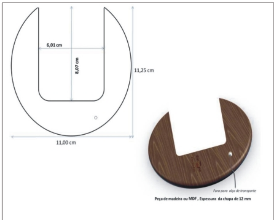
Figura 15 – Gabarito para conferir o diâmetro do tronco da árvore, utilizado em programa de desrama para a regulação da intensidade de sombra e produção de toras com alta qualidade de madeira (madeira sem nó).
